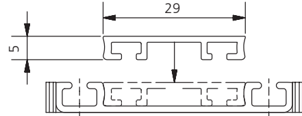
направляющая двойная + вставка (15.16.xx)
