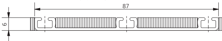
нижняя направляющая тройная (под заказ)
