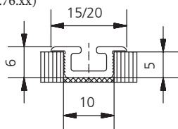
Нижняя направляющая одиночная врезная 15мм (14.76.xx)
