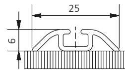
направляющая нижняя одиночная накладная (14.56.xx)
