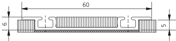
Внижняя направляющая двойная врезная 15.06.xx
