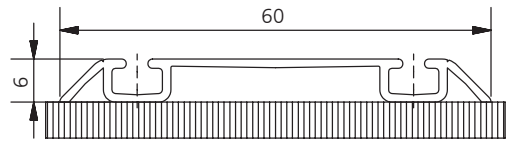
направляющая двойная + вставка (15.16.xx)
