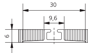
направляющая нижняя одиночная внутренняя (14.46.xx)
