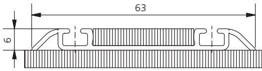
Внижняя направляющая двойная врезная (под заказ)
