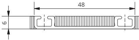
Внижняя направляющая двойная врезная 15.06.xx
